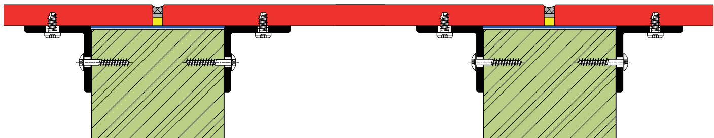
BALKONOVÁ PODLAHOVÁ DESKA UPEVNĚNÁ NA DŘEVĚNÉM TRÁMU (NEPŘÍZNANÉ UPEVNĚNÍ – ŠROUBEM)
