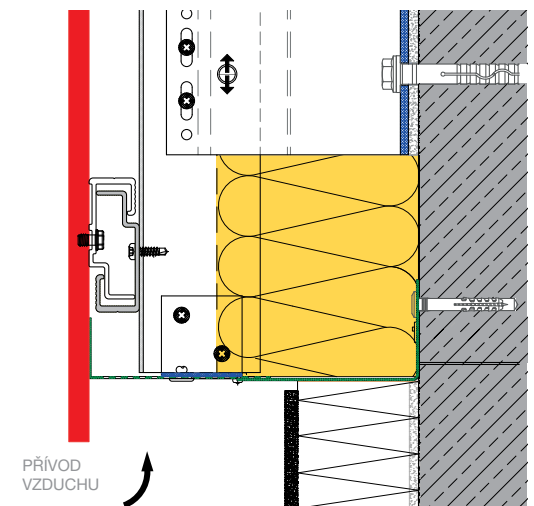
NAPOJENÍ NA PODEZDÍVKU A103
