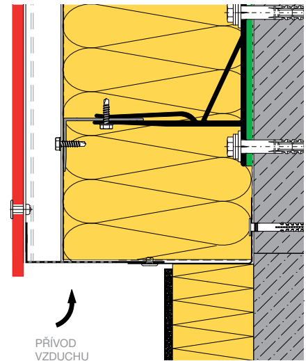
NAPOJENÍ NA PODEZDÍVKU A103
