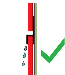
SVISLÝ ŘEZ
