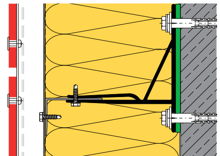
HORIZONTÁLNÍ SPÁRY A110
