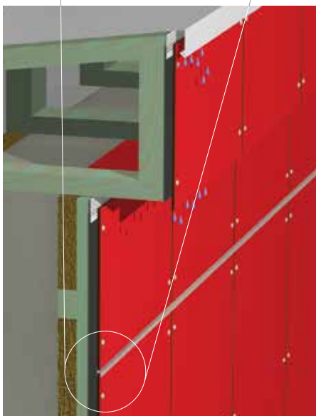
OCHRANA PROTI DEŽI V OBLASTI ATKY/ ZAKONČENÍ STŘECHY
