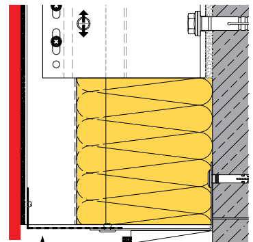
NAPOJENÍ NA PODEZDÍVKU A103
