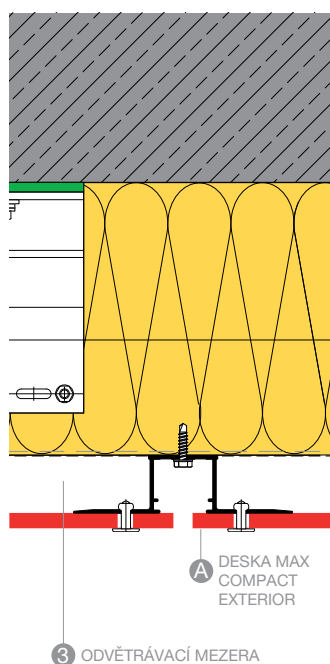
SVISLÁ SPÁRA A107
