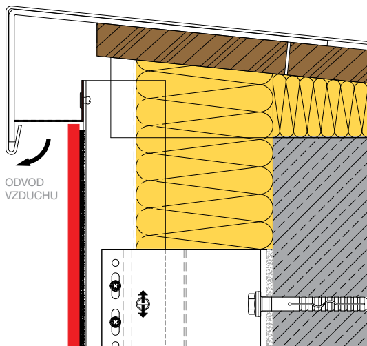
STŘEŠNÍ NAPOJENÍ - ATIKA A109
