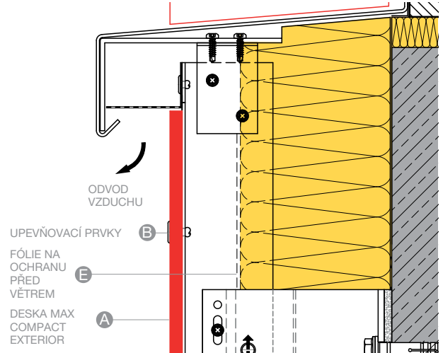
NAPOJENÍ PARAPETU A102
