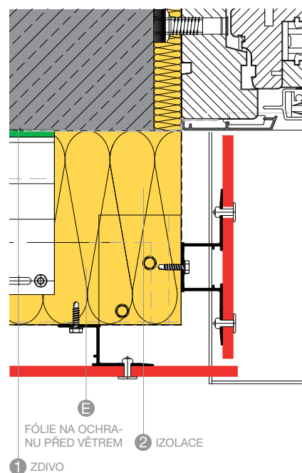
OKENNÍ OSTĚNÍ (ŠPALETA) A104
