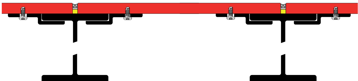
BALKONOVÁ PODLAHOVÁ DESKA UPEVNĚNÁ NA OCELOVÉM NOSNÍKU (NEPŘÍZNANÉ UPEVNĚNÍ – ŠROUBEM)
