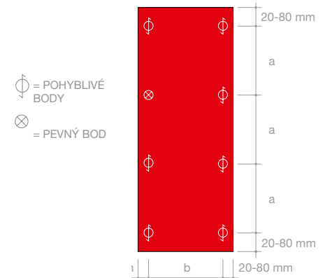
DESKA S JEDNÍM POLEM
