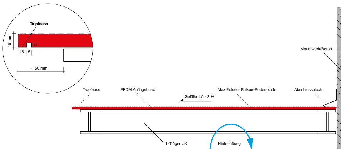
PRINCIP KOLMÉHO ŘEZU ODVĚTRÁVÁNÍ ZE ZADU A SKLONU
